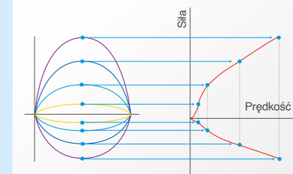
Wykres ze stanowiska kontrolnego: test mający na celu ocenę siły tłumienia w funkcji prędkości ruchu tłoka amortyzatora.
